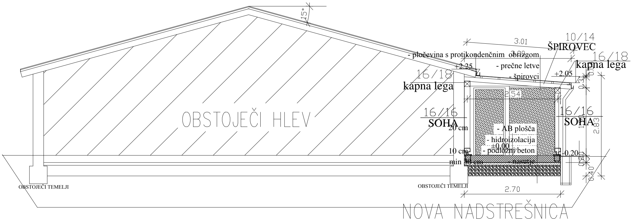
PREREZ A-A
